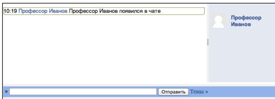
Рис. 6 – Окно чата
